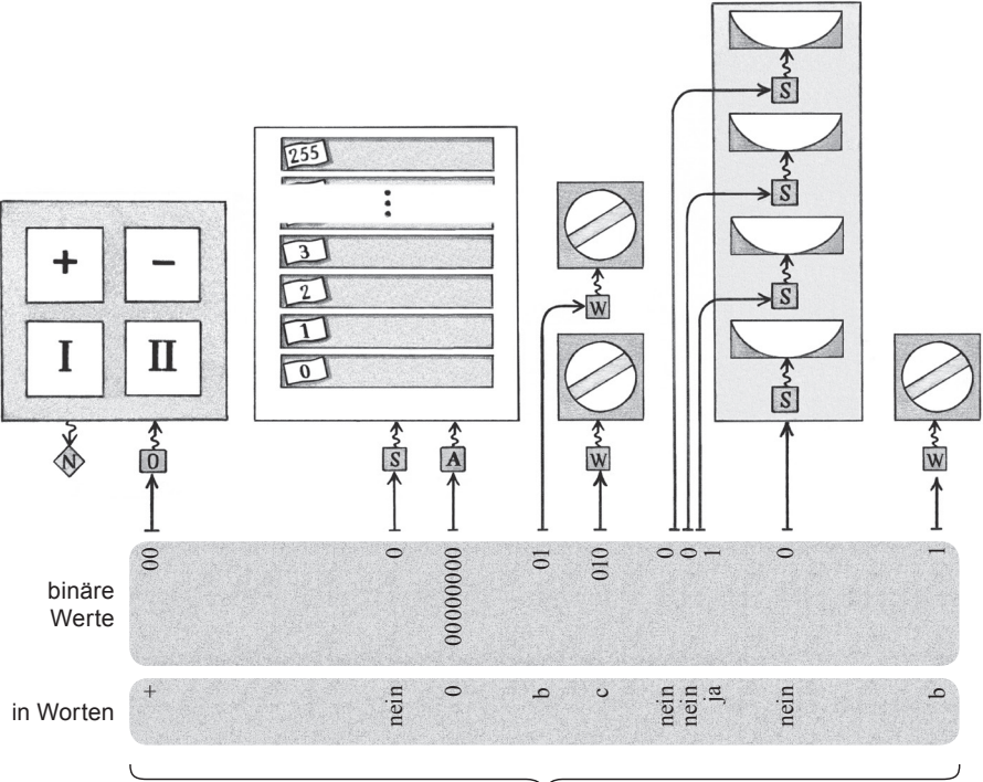
Steuerleitungsbelegung
