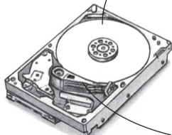
Festplatte
