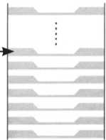
Hauptspeicher
